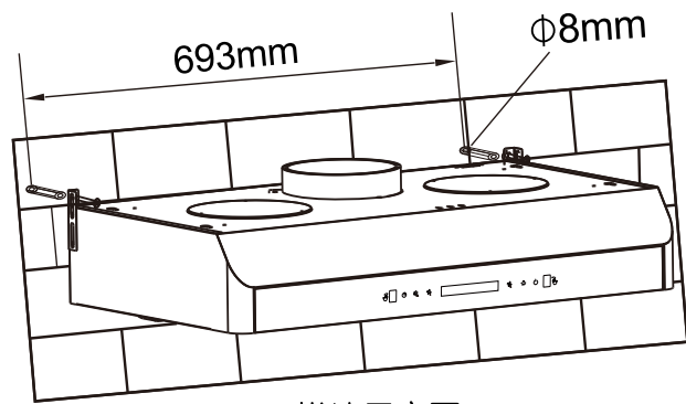
掛牆示意圖
