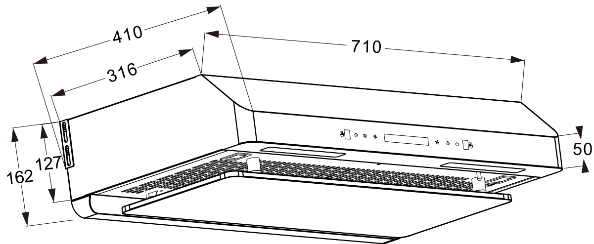
整機尺寸圖(mm)
