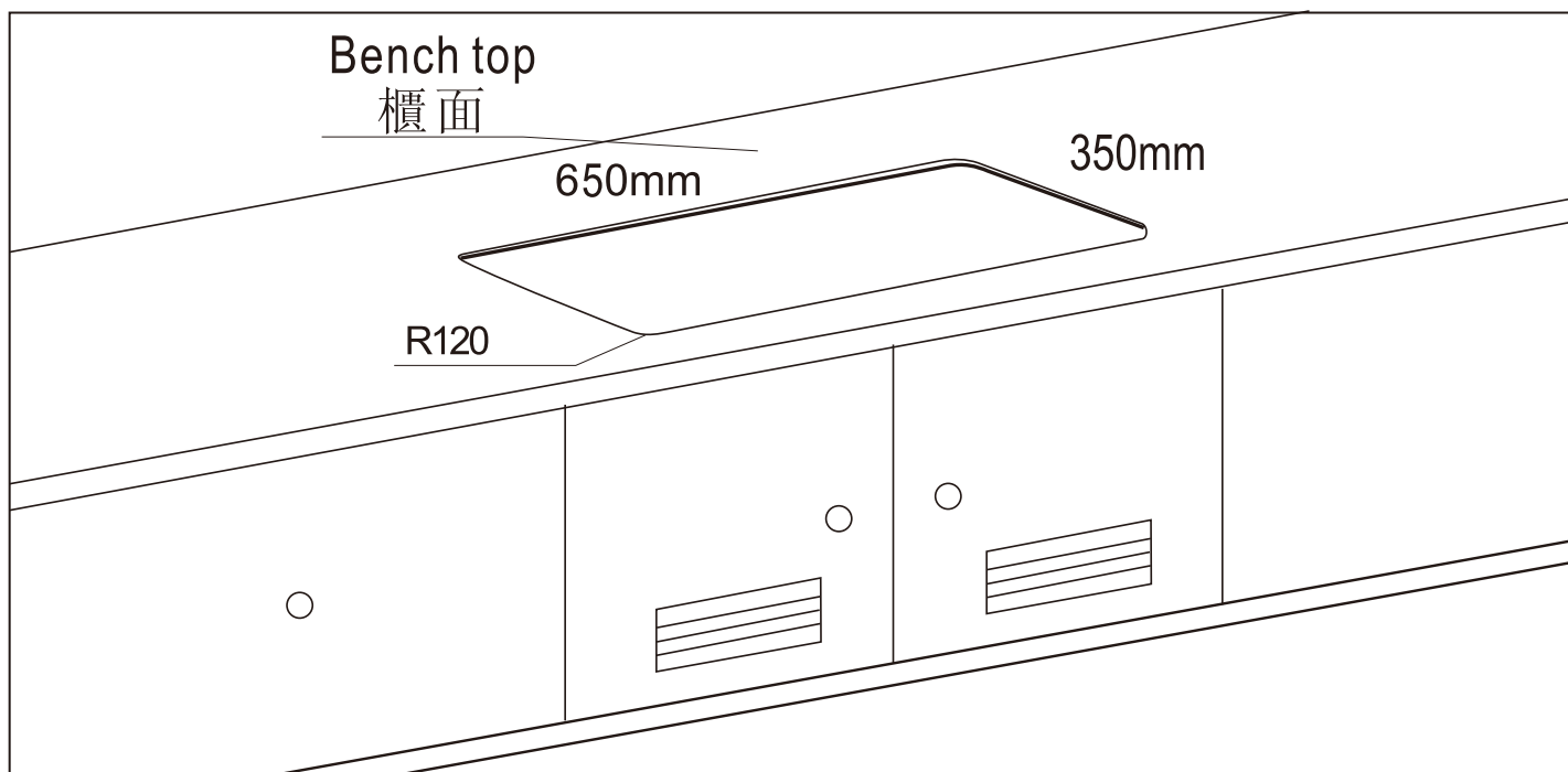
櫃面開孔尺寸
