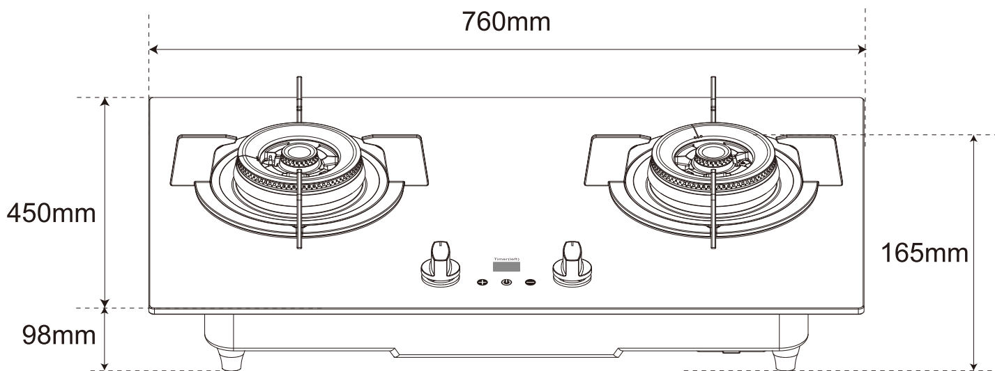
機身尺寸
