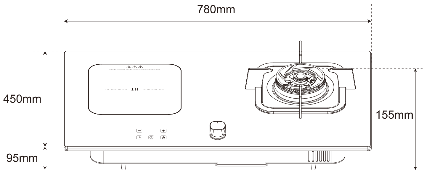
機身尺寸
