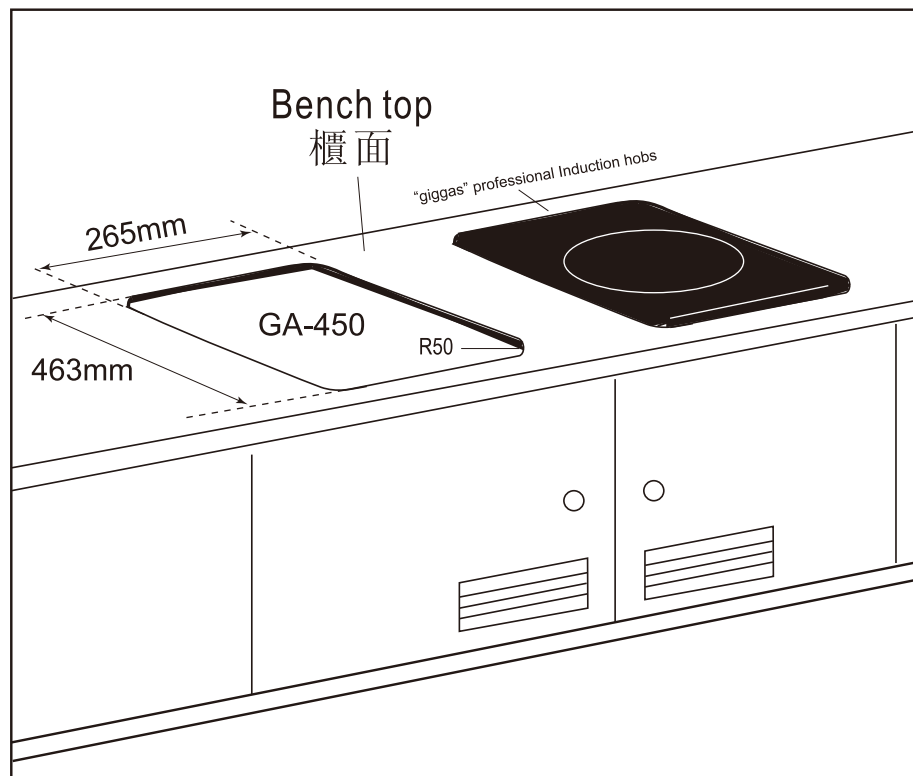
櫃面開孔尺寸
