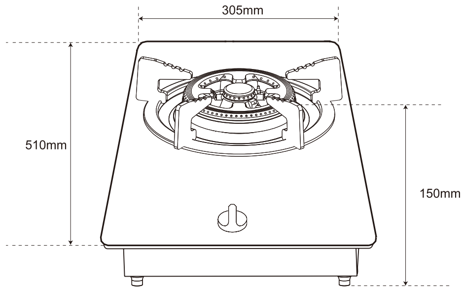
機身尺寸
