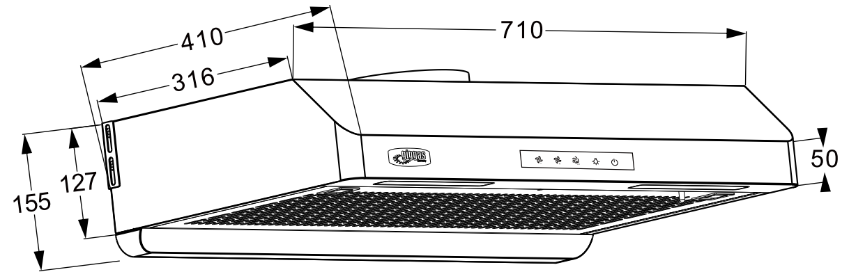
整機尺寸圖(mm)
